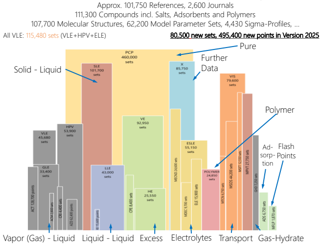
Status of the Dortmund Data Bank (Version 2025)
